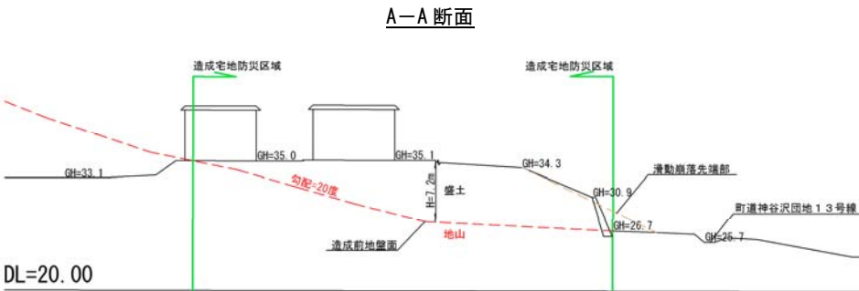
神谷沢宅地滑動崩落対策事業（断面図）
