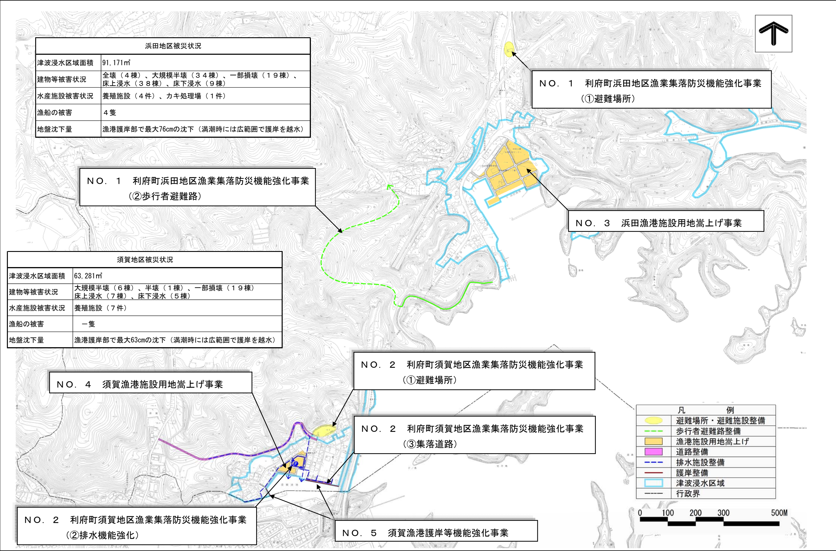
復興交付金事業位置図（４）（浜田・須賀地区）【県事業分】
