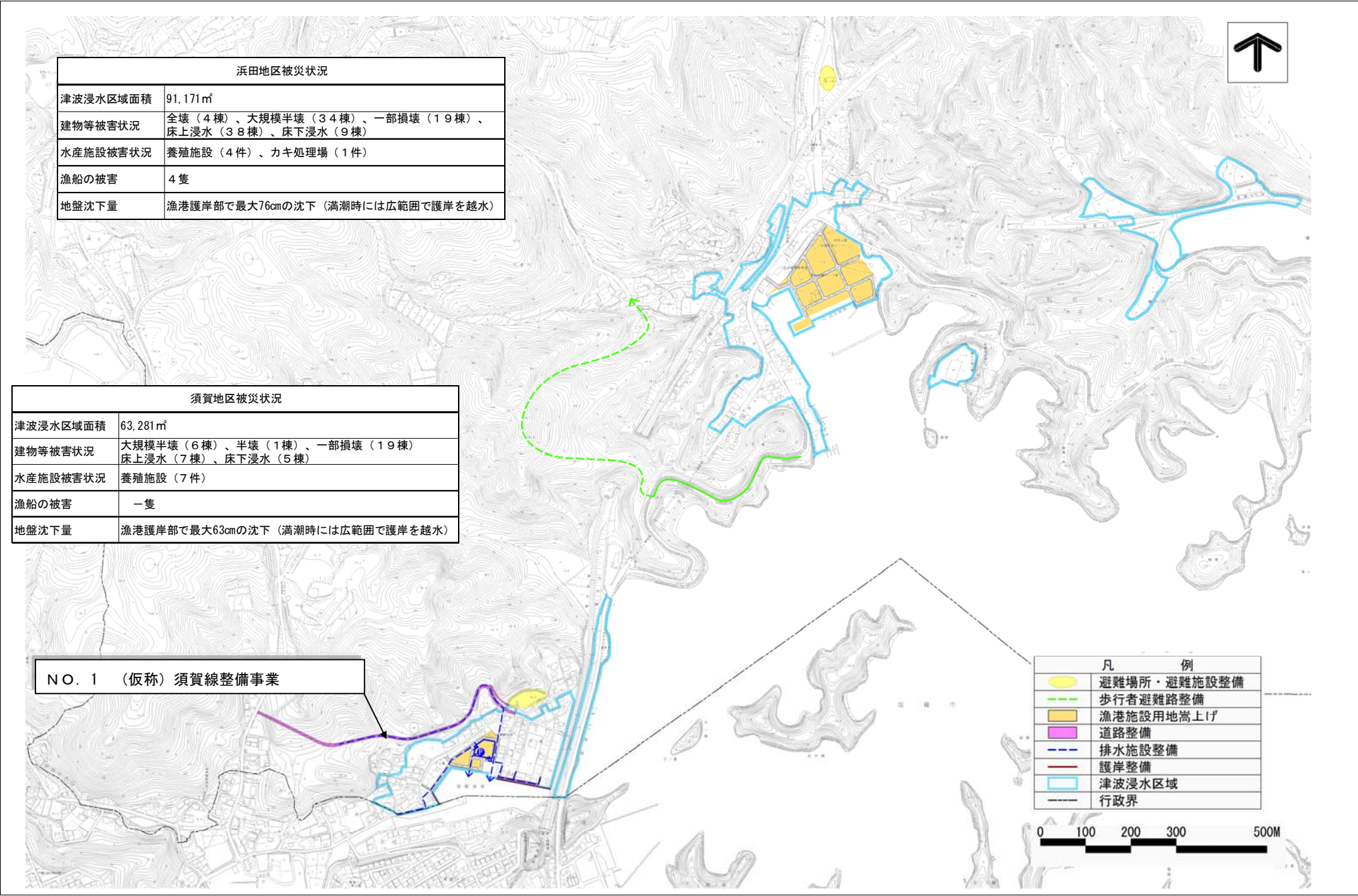
復興交付金事業位置図（２）（浜田・須賀地区）【町事業分】
